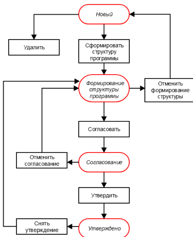
Рисунок 11 – Блок-схема статусной модели ЭД «Государственная программа/Подпрограмма/Основное мероприятие»
